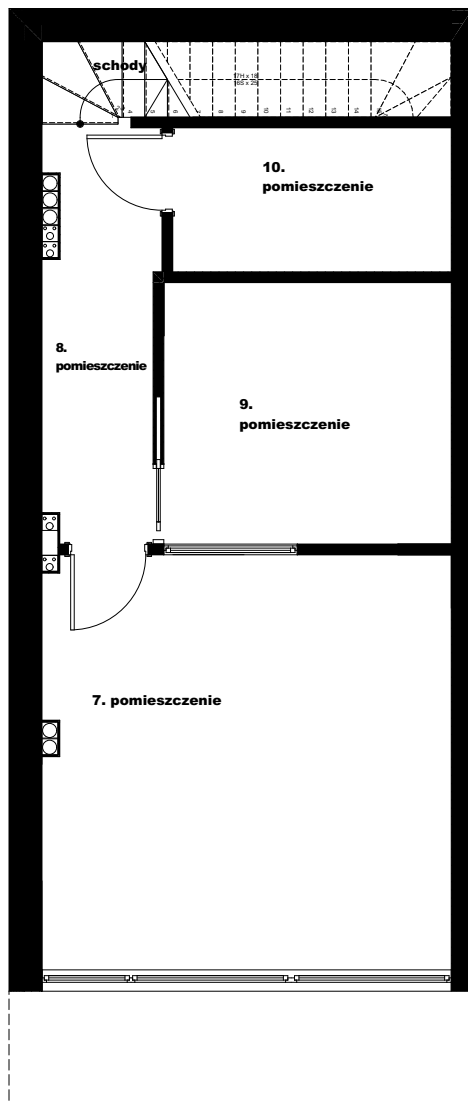
poziom lokalu 0
